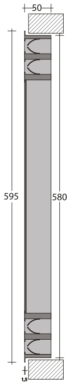
[ img,1 corte vertical ]
