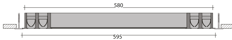
[ img,3 corte horizontal com difusor apoiado nos perfis do tecto modular em substituição de uma placa ]
